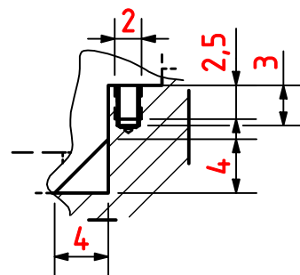
DETALLE D (2 : 1)
