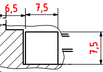
DETALLE C (2 : 1)
